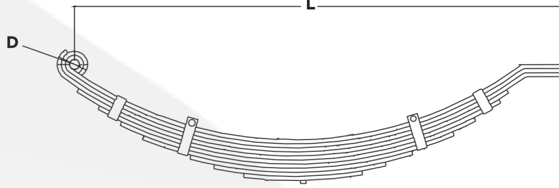
TEKNİK ÇİZİM
